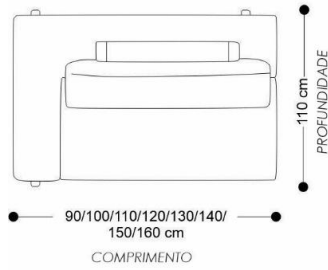
MÓDULO FIXO COM BRAÇO
