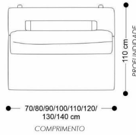
MÓDULO FIXO SEM BRAÇO
