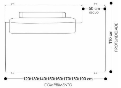
MÓDULO SEM BRAÇO COM RECUO
